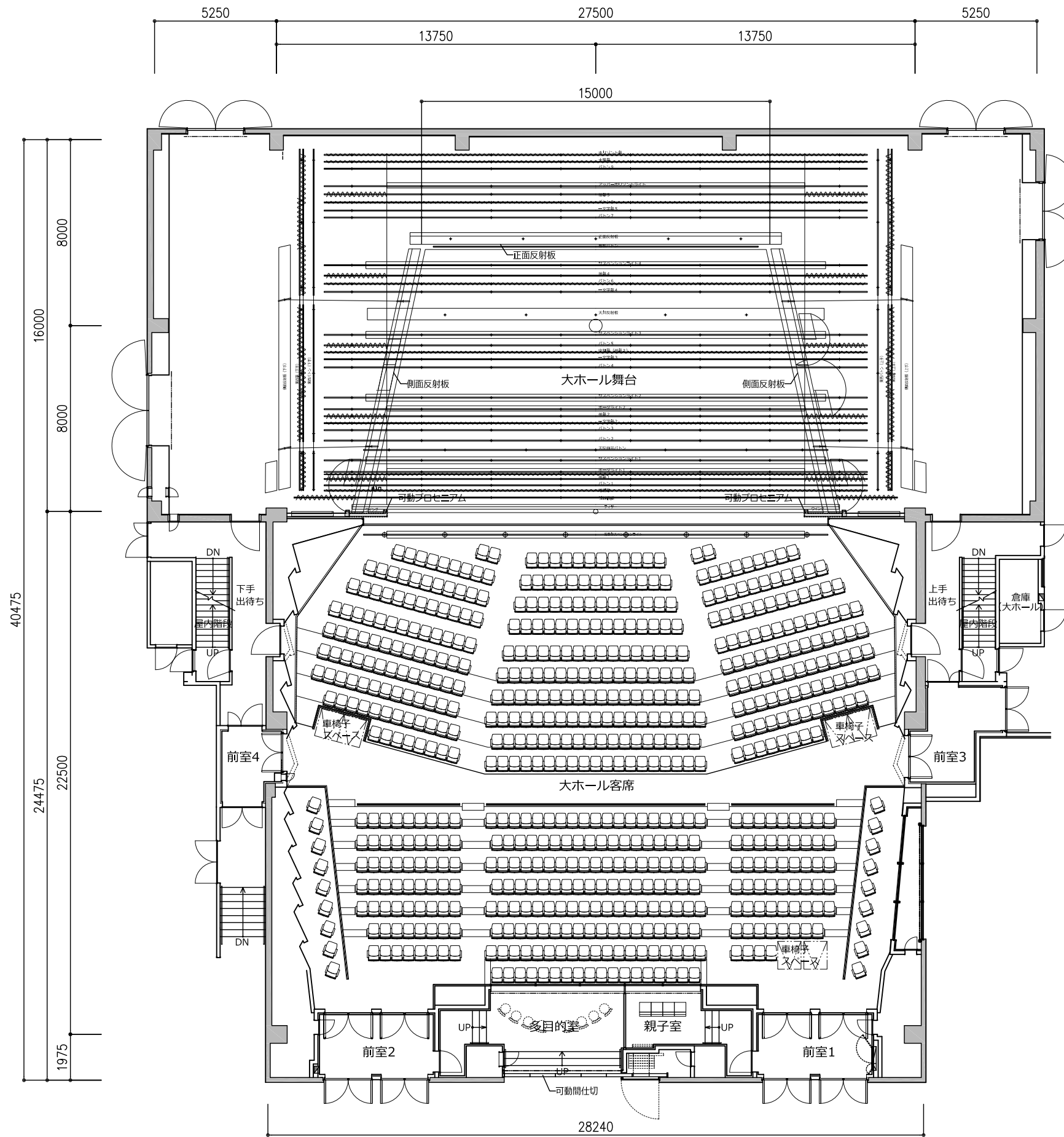
大ホール全体図 (1階) S=1/200 (A3)
