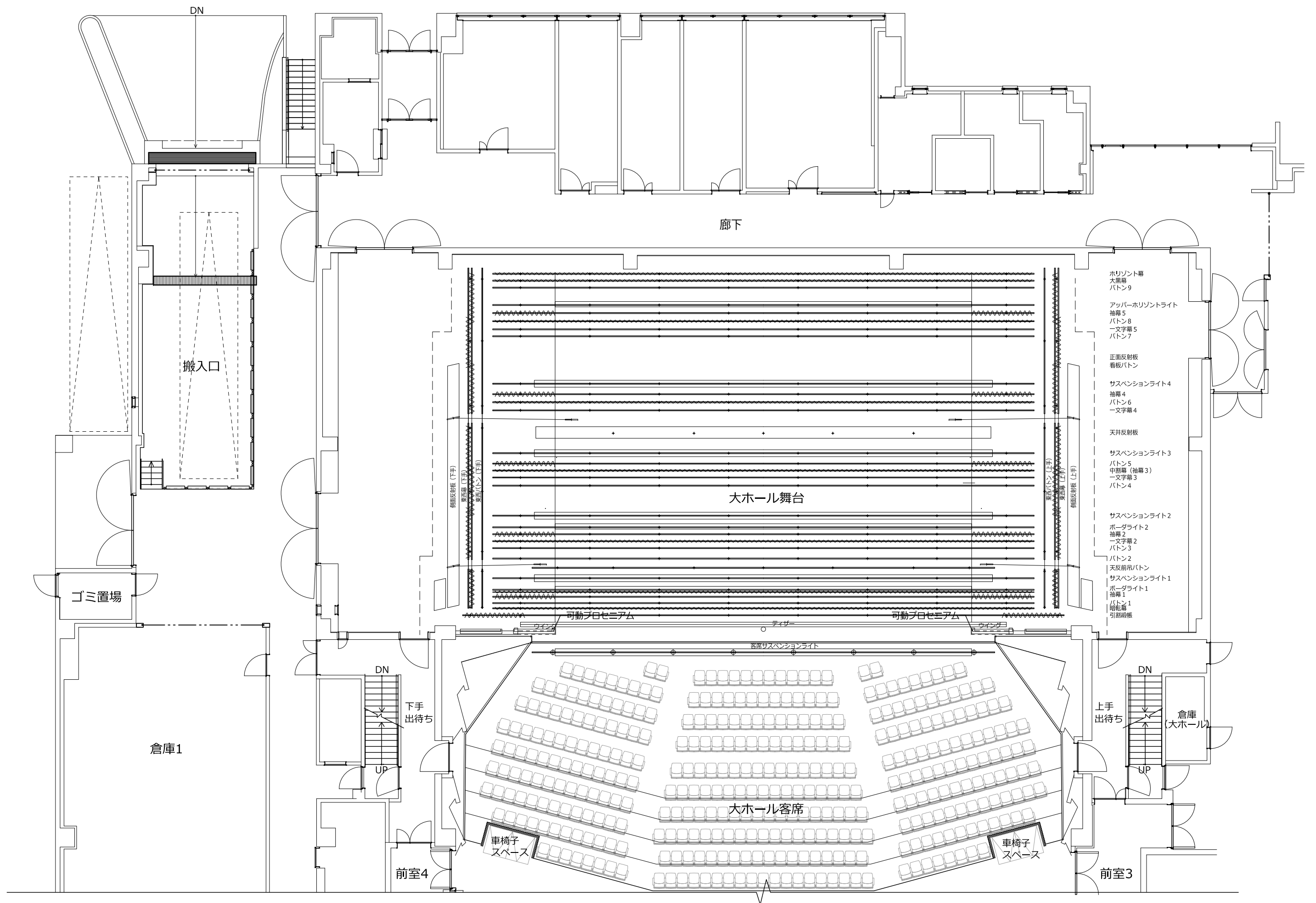
大ホール舞台平面図 (上層) S=1/150 (A3)
