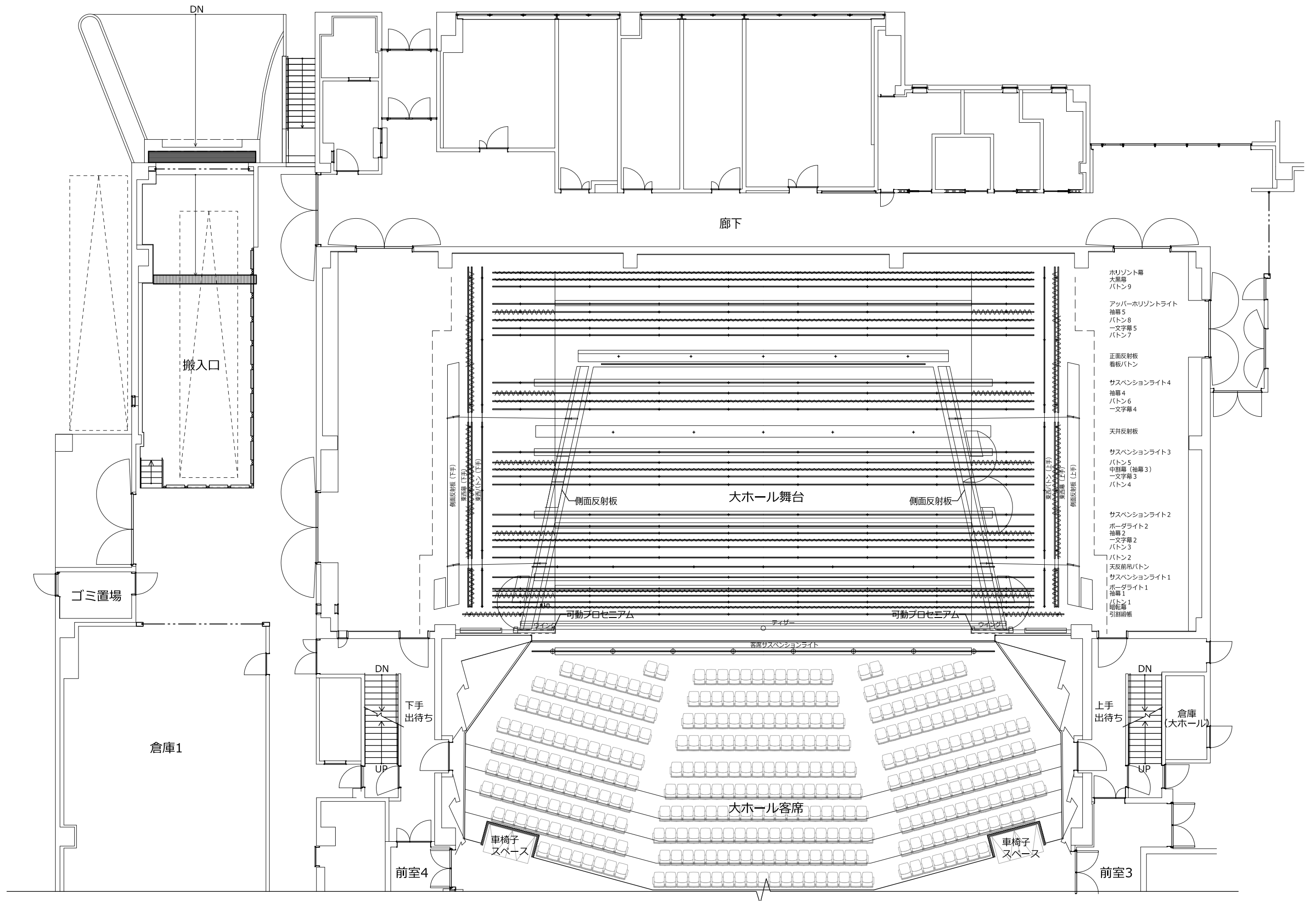
大ホール舞台平面図 S=1/150 (A3)
