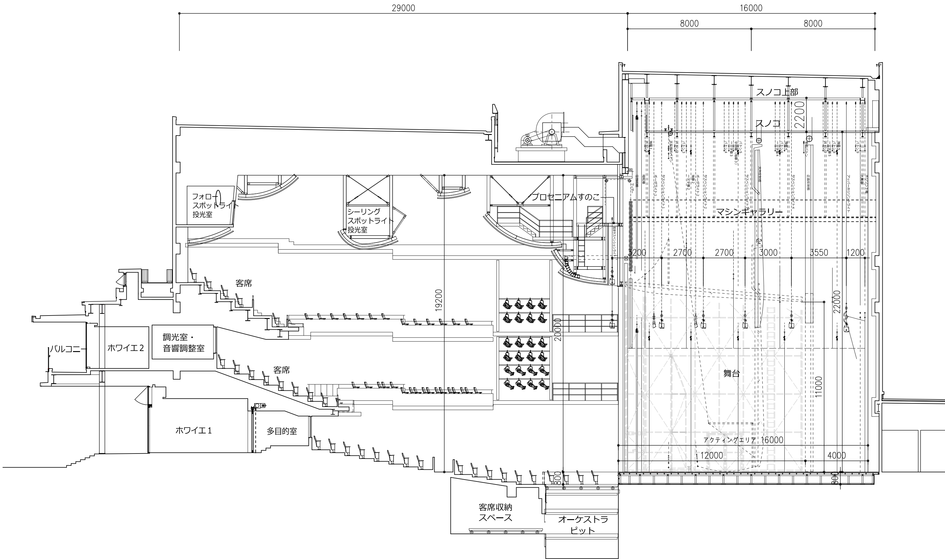
大ホール舞台断面図 S=1/150 (A3)
